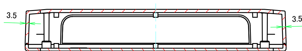
B-B ( 1 : 2.5 )
