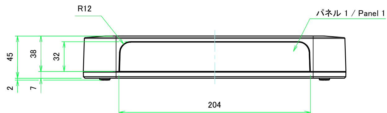
B-B ( 1 : 2.5 )
